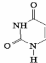
Ураци́л (У)
