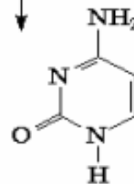
Цитозин (Ц)
