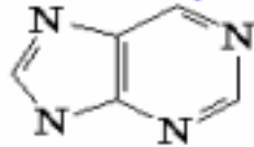
пури́н
