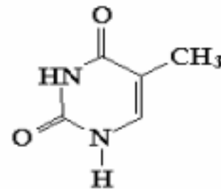
Тими́н (Т)
