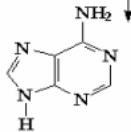
Аде́нин (А)
