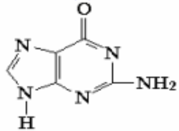
Гуа́нин (Г)
