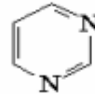
пири́мидин
